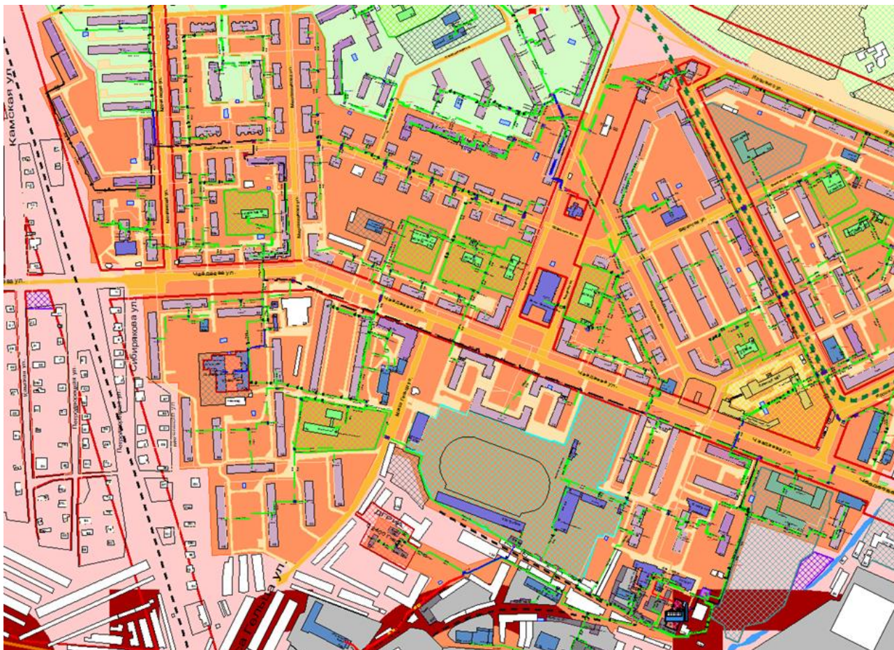
Рисунок 3.99 – Трассировка теплопровода от котельной ОАО «Нижегородский авиастроительный завод «Сокол» по ул. Чаадаева, д. 10 до конечного потребителя «ПТ-Мечн,63»
